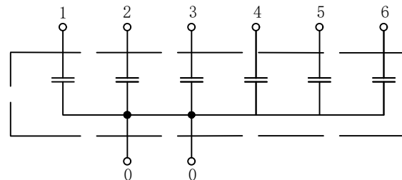
电热电容器基本参数
